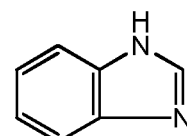
benzimidazole
