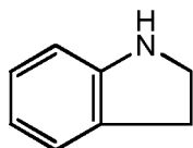
indoline
