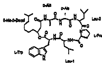
Kahalalide E (5)
