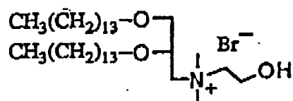
DMRIE
