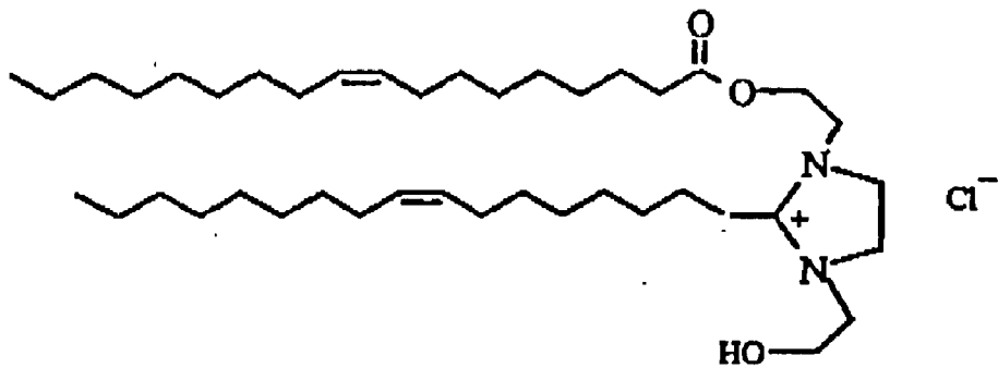
DOTIM
