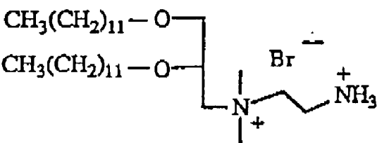
GAP-DLRIE
