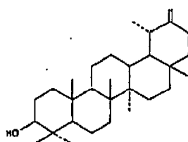
Taraxasterol (taraxastanes)
