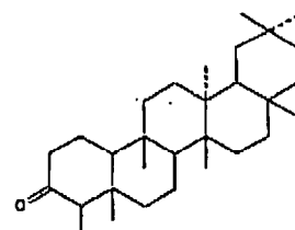
Friedelin (friedelanes)
