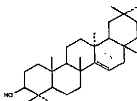
Taraxerol (taraxeranes)
