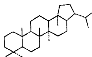
(Hopanes)
