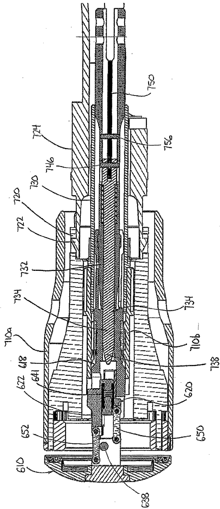
FIG. 73
