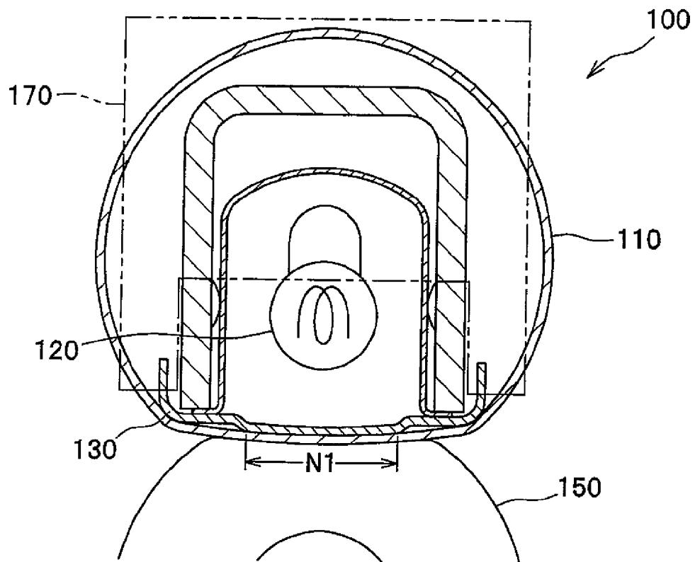
Fig.10A
