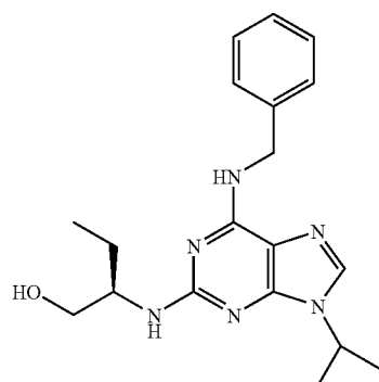
Roscovitine
