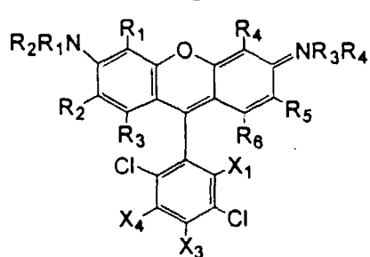
4,7-Dichlororhodamine
