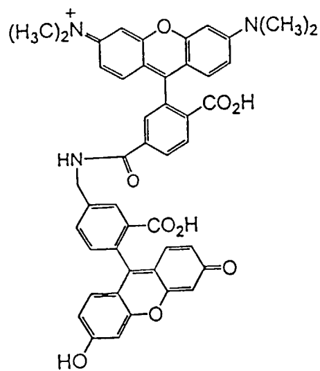
6-TMR-5AMF
