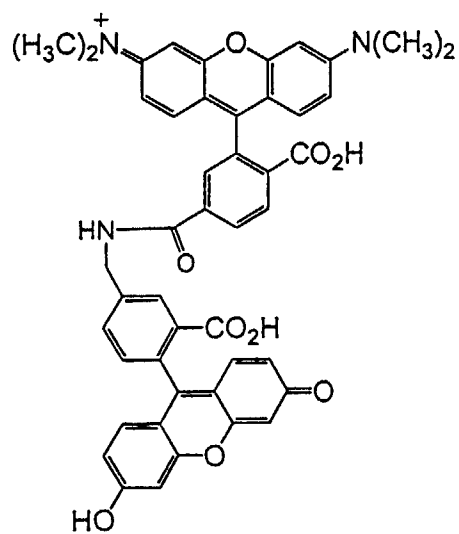
6-TMR-5AMF
