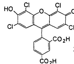
TET
