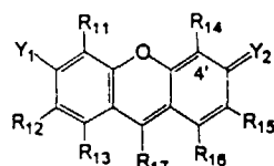
XANTHENE
