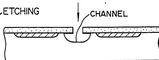
FIG. 8D THERMAL OXIDATION
