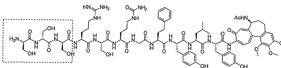
NH 2 -D-Ser-D-Ser-D-Ser-Arg-Ser-Cit-Gly-HoPhe-Tyr-Leu-Tyr-Warhead
