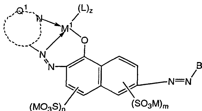
Formule générale (IV-1)
