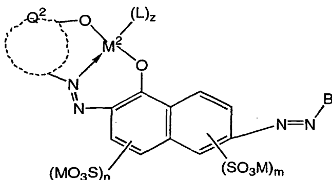
Formule générale (IV-2)
