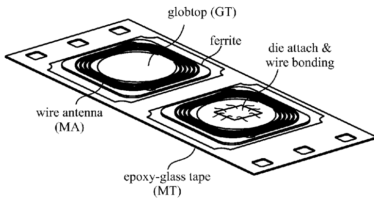
FIG.6D DIF Module
