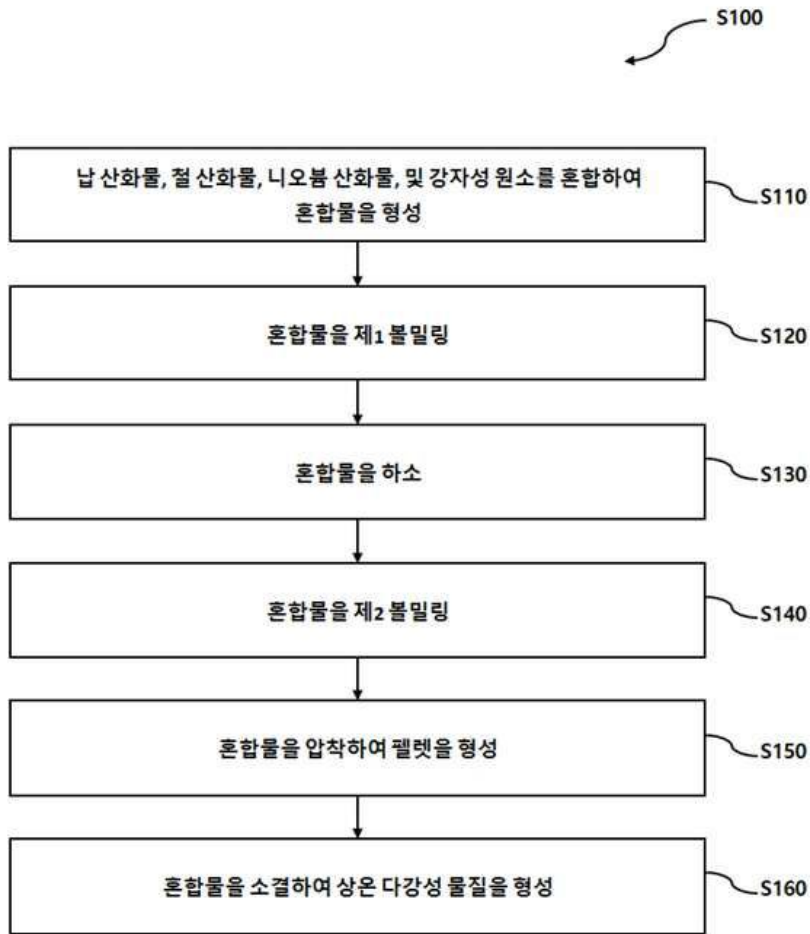
도면2
