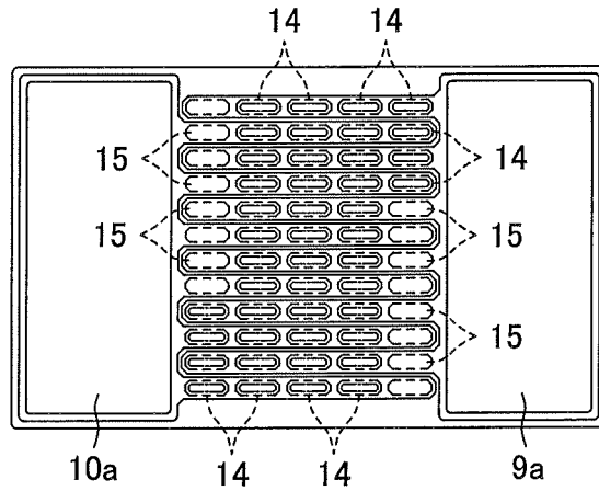
FIG. 7E Arrangement Example 5
