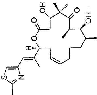
desoxyepothilone A
