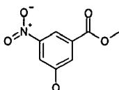
Compound (d)
