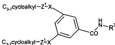
Formula (IIk)
