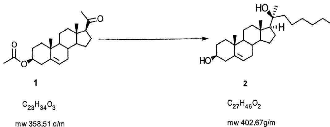
Pregnenolone acetate
