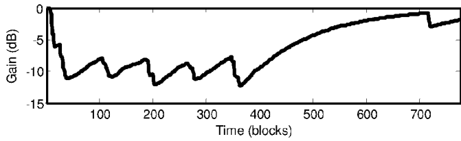
FIG. 10b b) DRC gain
