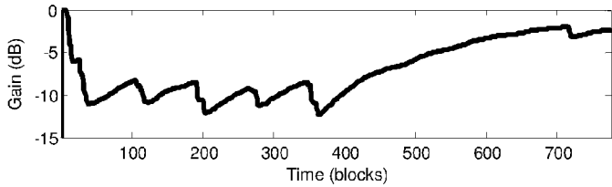
FIG. 10e e) Event-controlled DRC gain
