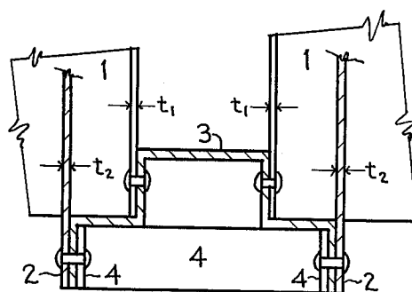
SECTION B-B FIG. 1
