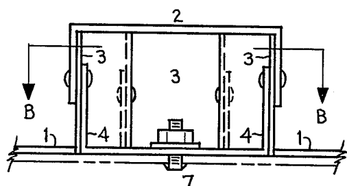
VIEW A-A FIG. 2
