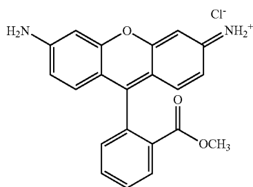
Rhodamine 123
