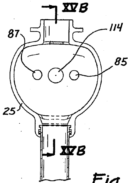
Fig. 13A
