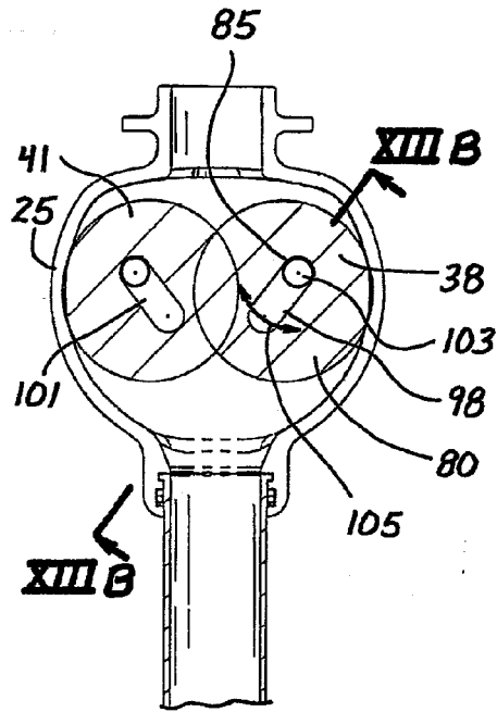
Fig. 13A
