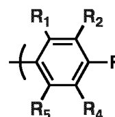
(IIg)
