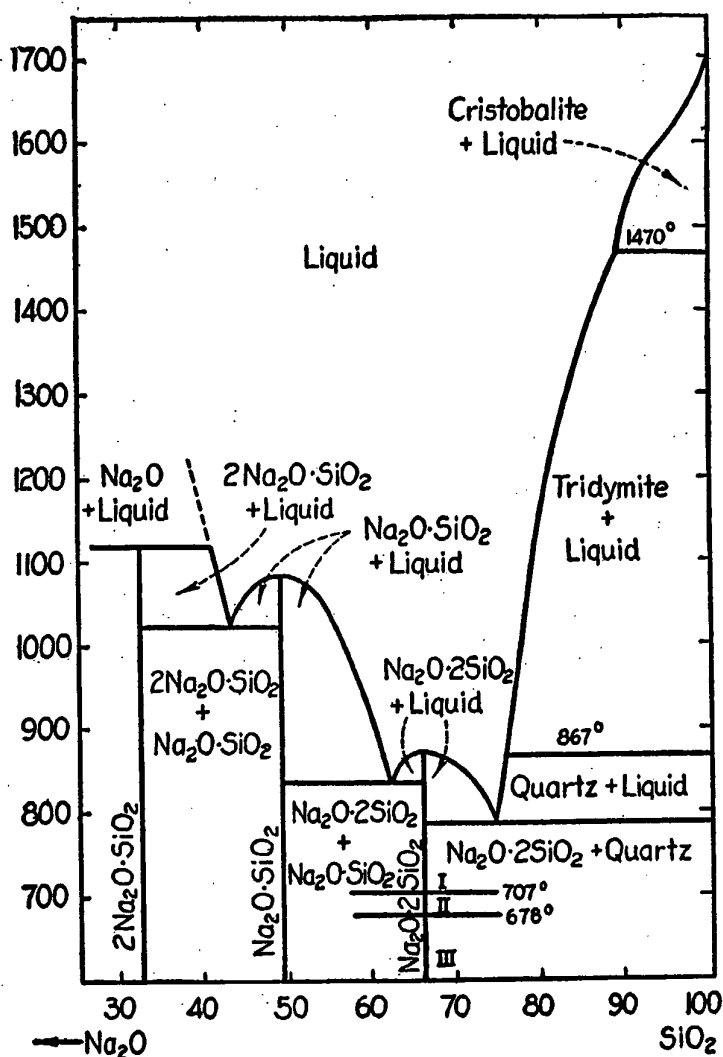
FIG. 192.—System \text{SiO}_2-2\text{Na}_2\text{O} \cdot \text{SiO}_2 .
