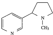
nicotine
