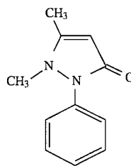
antipyrine
