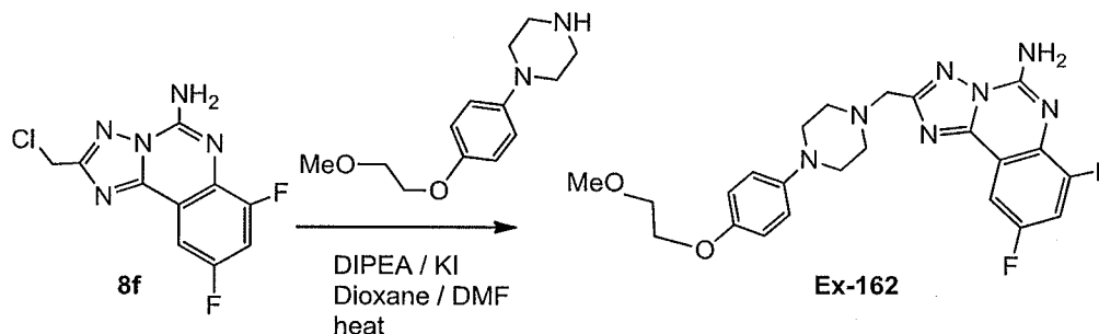
Scheme E3-ac
