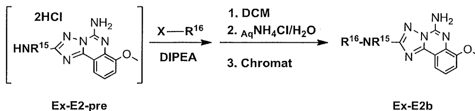
Scheme E1
