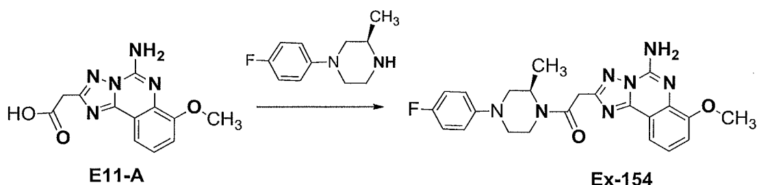
Scheme E11
