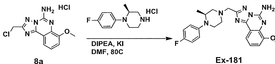
Scheme E2
