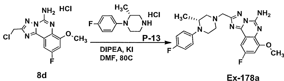
Scheme E3
