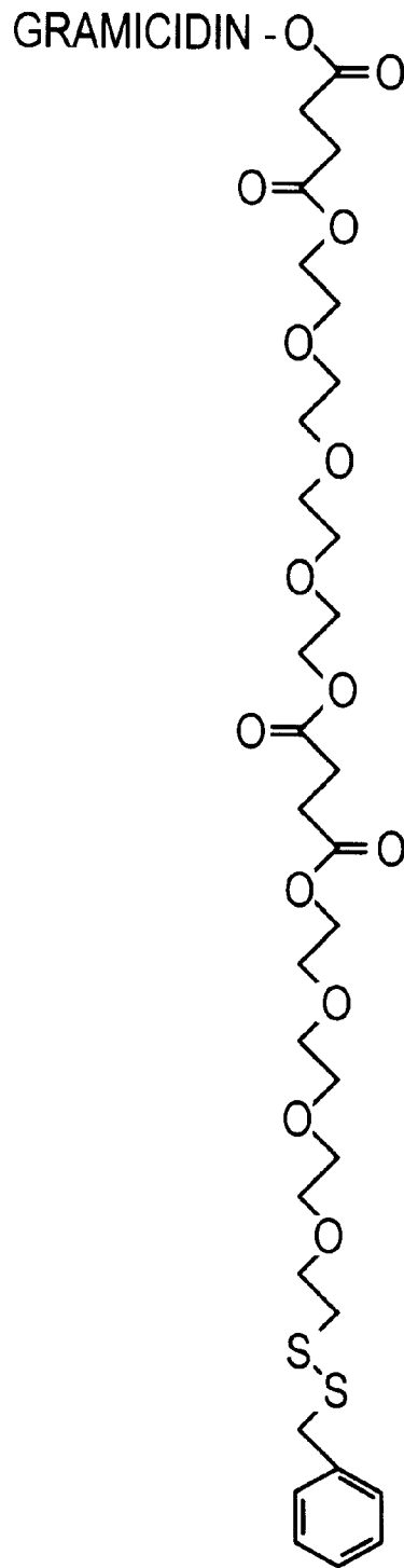
LINKER GRAMICIDIN E
