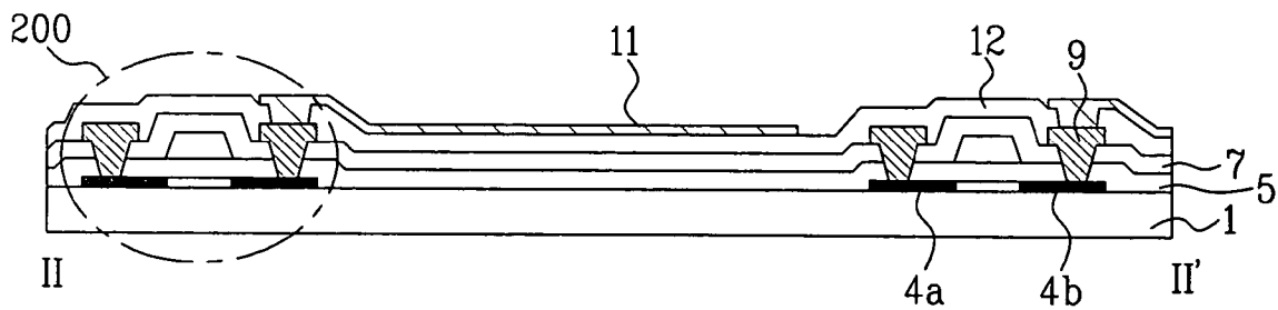
FIG. 2C
