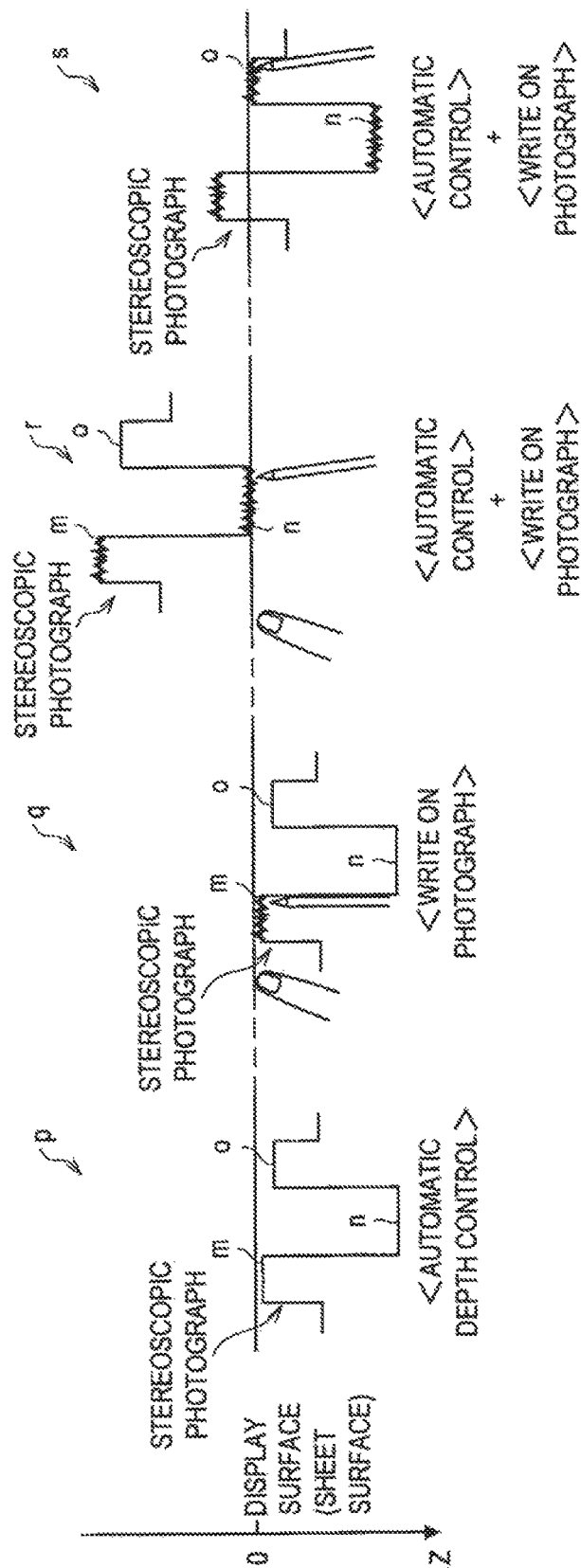
FIG. 17
