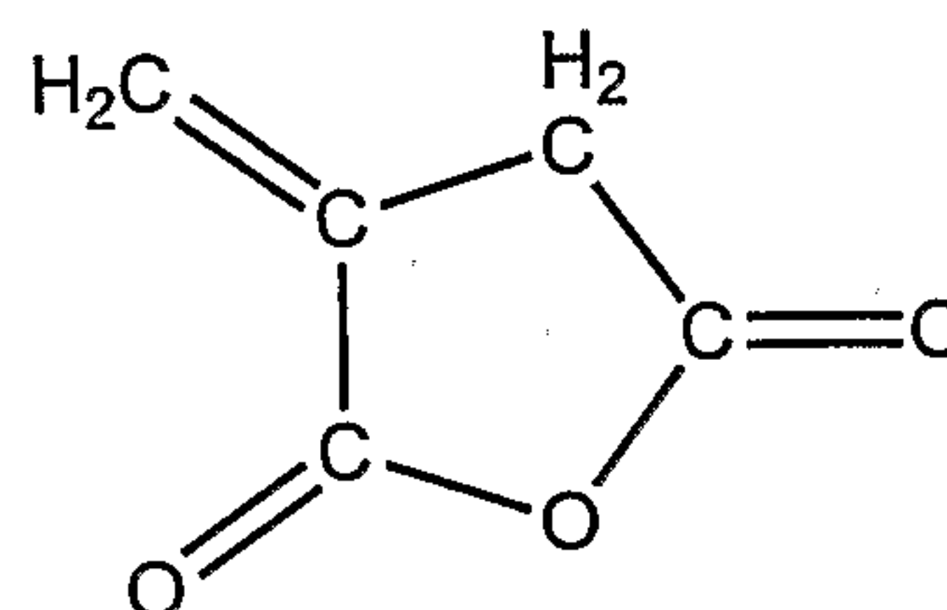
Itaconic Anhydride
