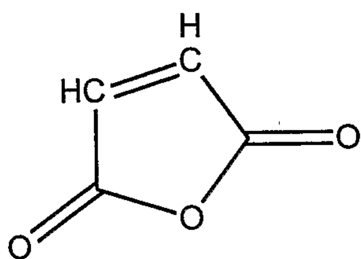
Maleic Anhydride
