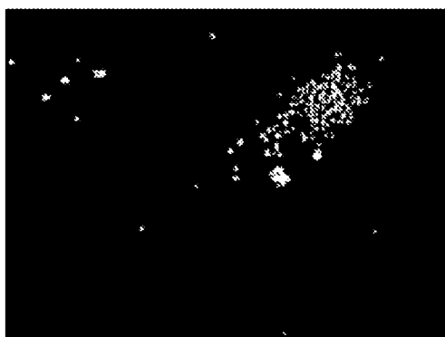
beta-D-amino-LNA; 2752
