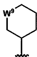
(1b-5)
