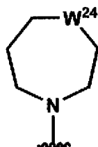
(1b-14)
