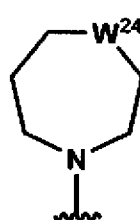
(1b-14)
