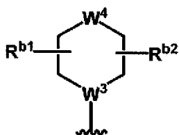
(1b-2)
