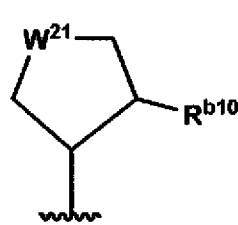
(1b-11)
