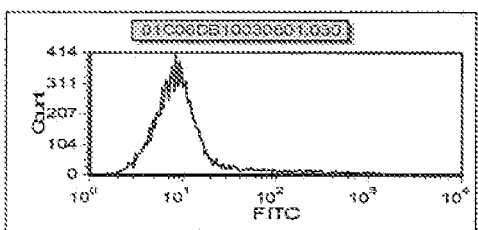
CRLR: RAMP1 Q28-A34
