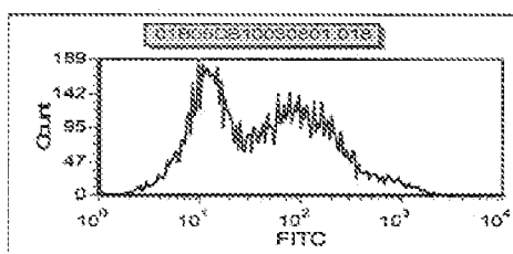
CRLR: RAMP1 Wild Type
