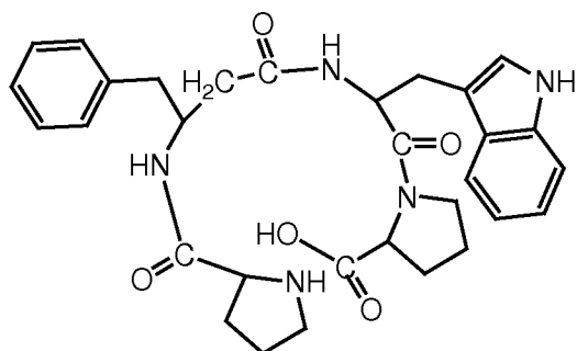
II-4-d ( \text{H-Pro-Pro-}\beta^3\text{hoPhe-Trp-OH} ),
