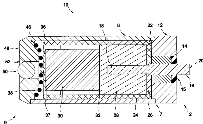
A - A
