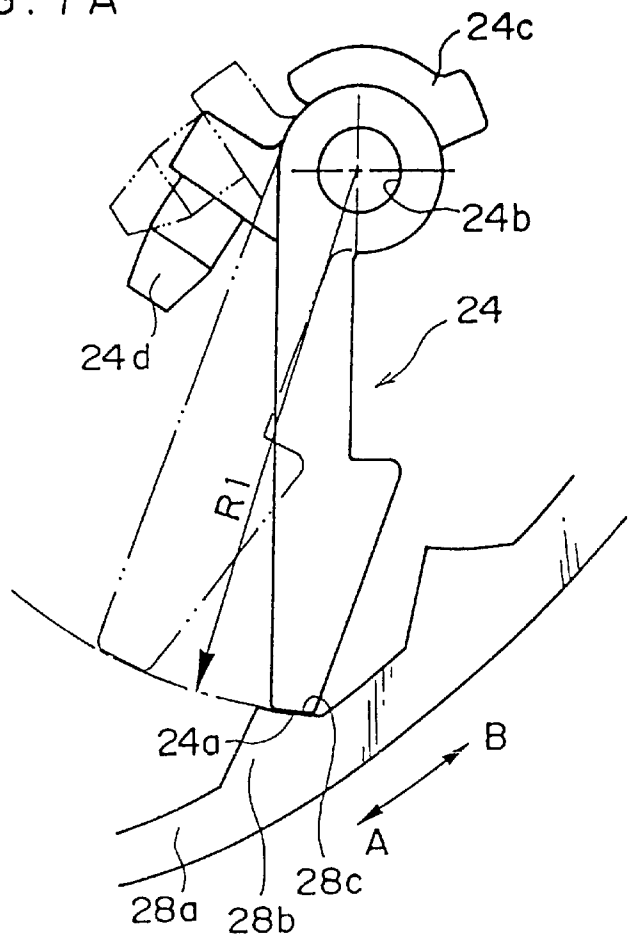
FIG. 7A
