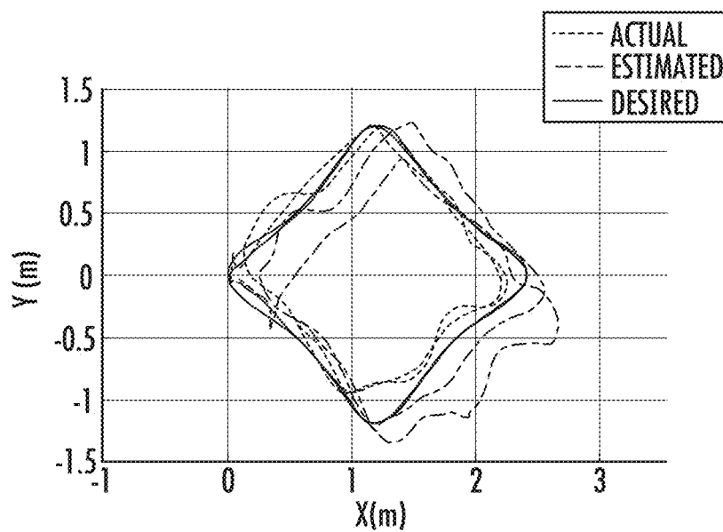
DESIRED, ESTIMATED, AND ACTUAL TRAJECTORIES
