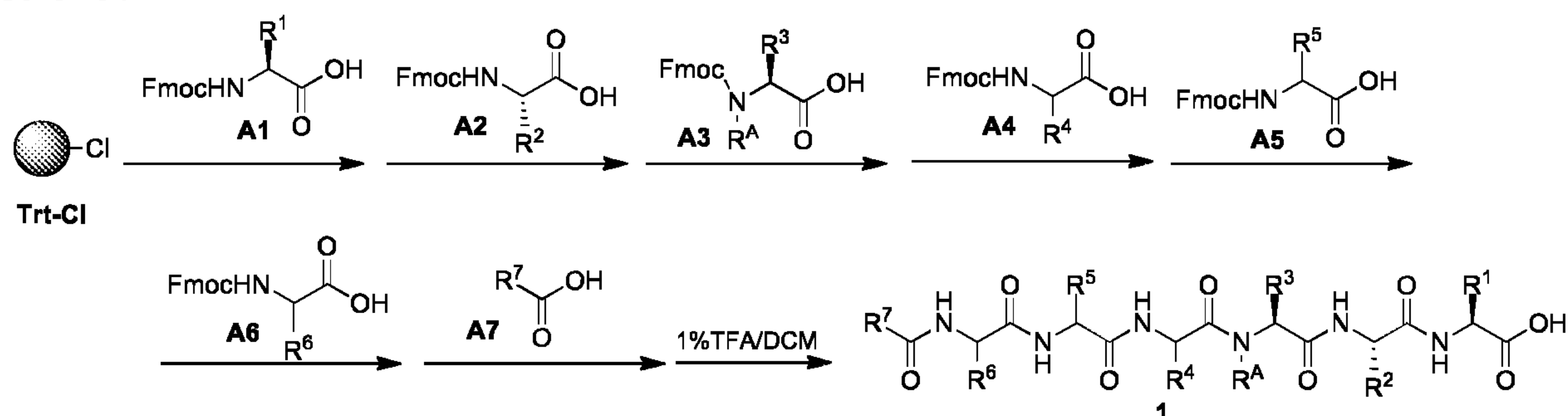
Scheme 1A
