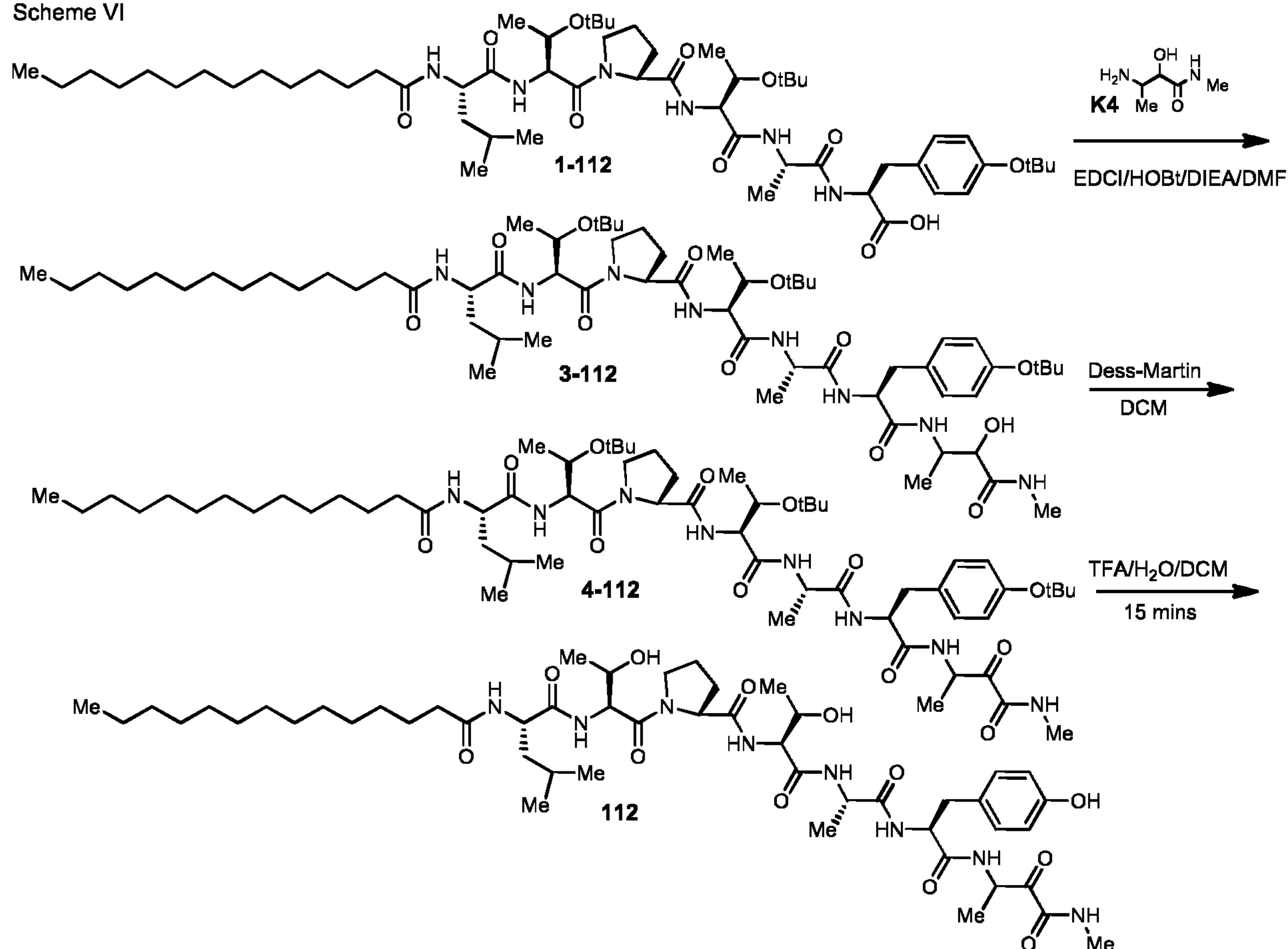
Scheme VI
