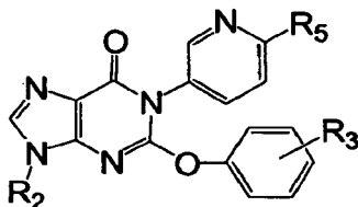
Formula Va
