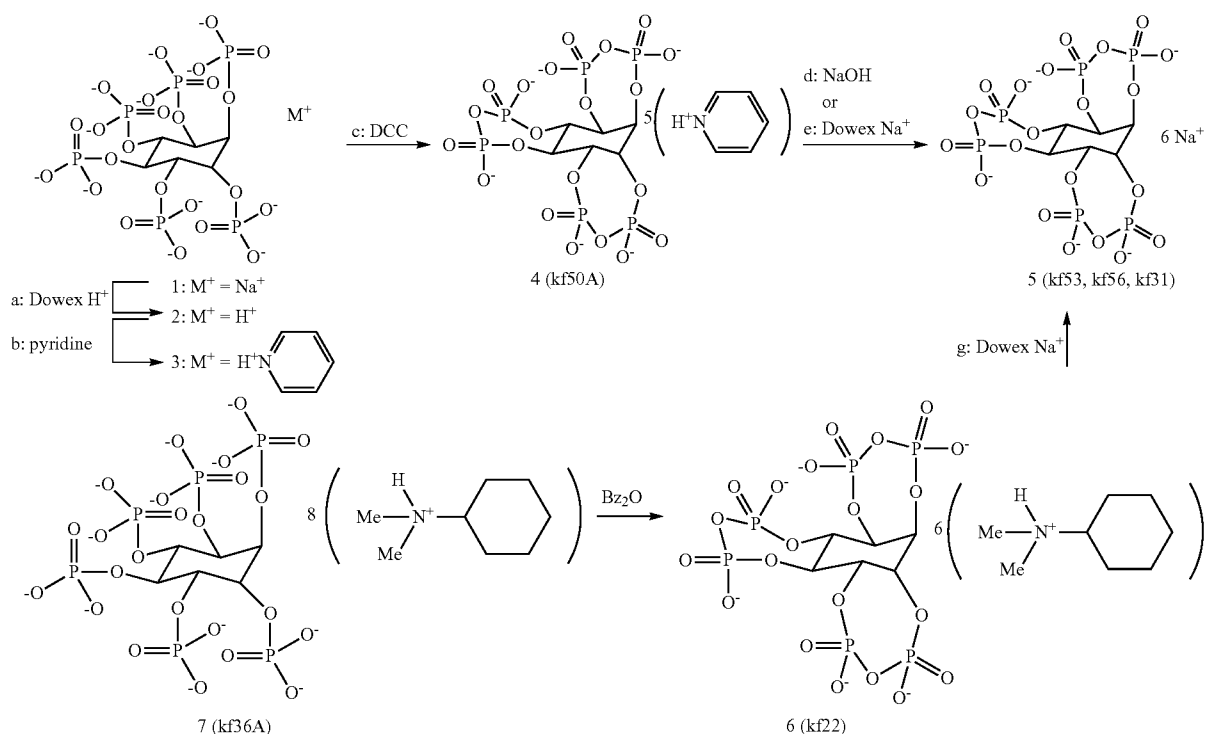
Scheme 3. The ITTP Na salts formation
