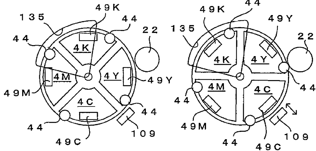
FIG. 5A : HOME POSITION
