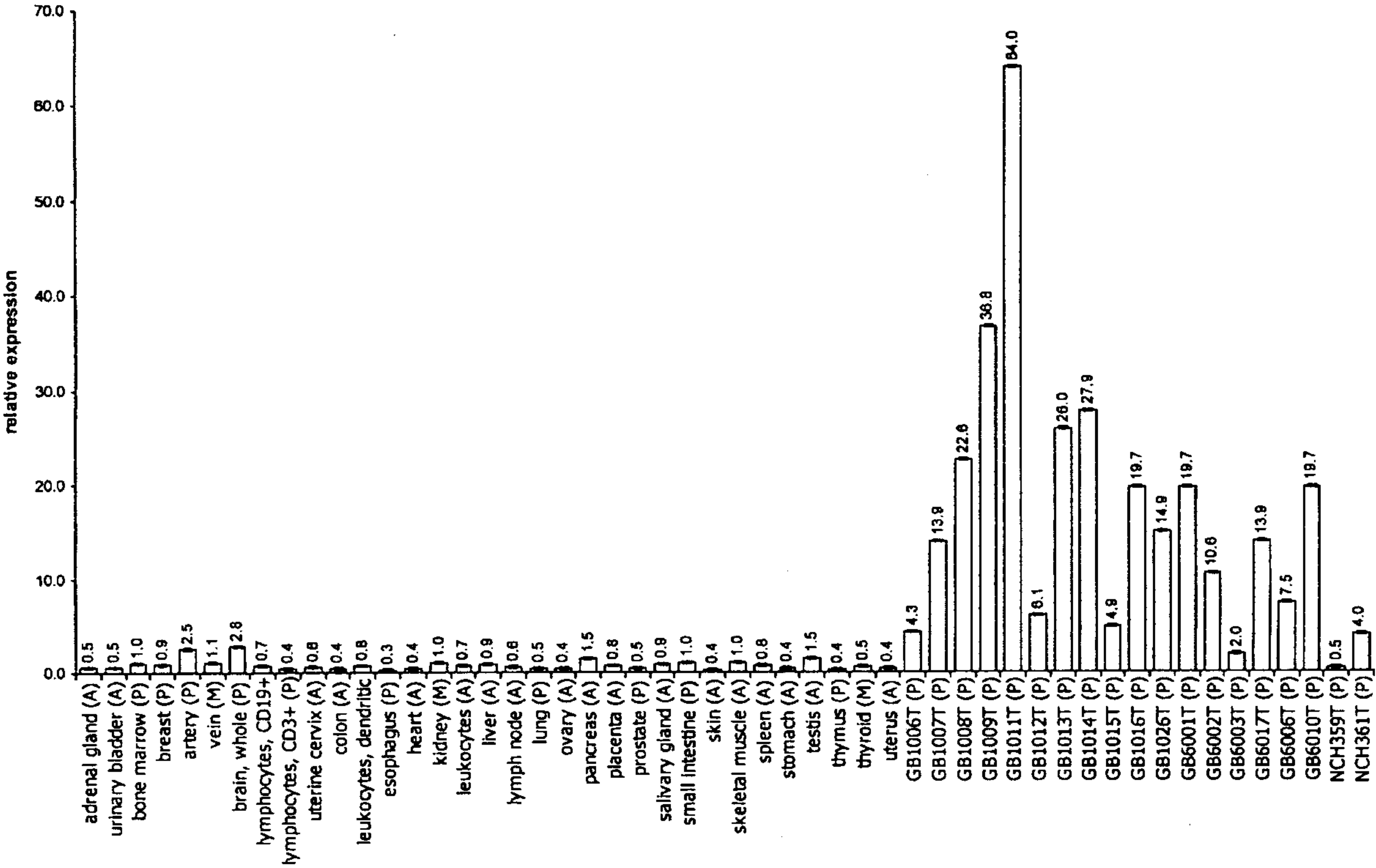
a) SLCO1C1 (Probeset ID: 220460_at)
