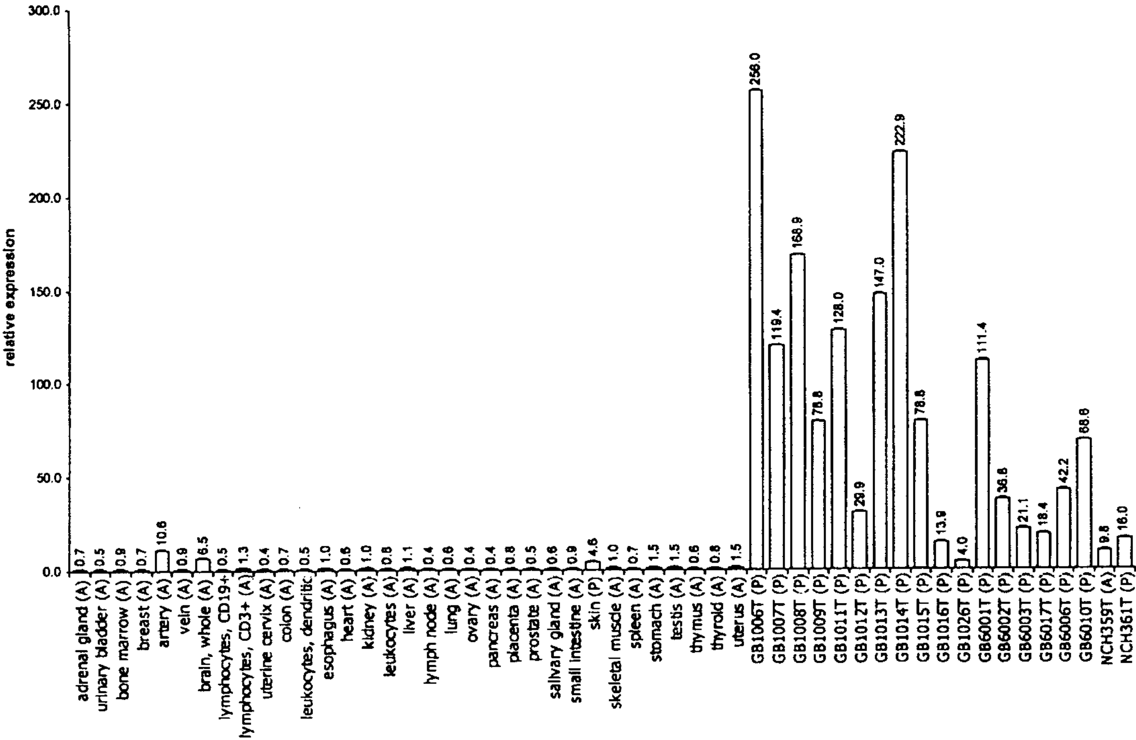
b) NR2E1 (Probeset ID: 207443_at)
