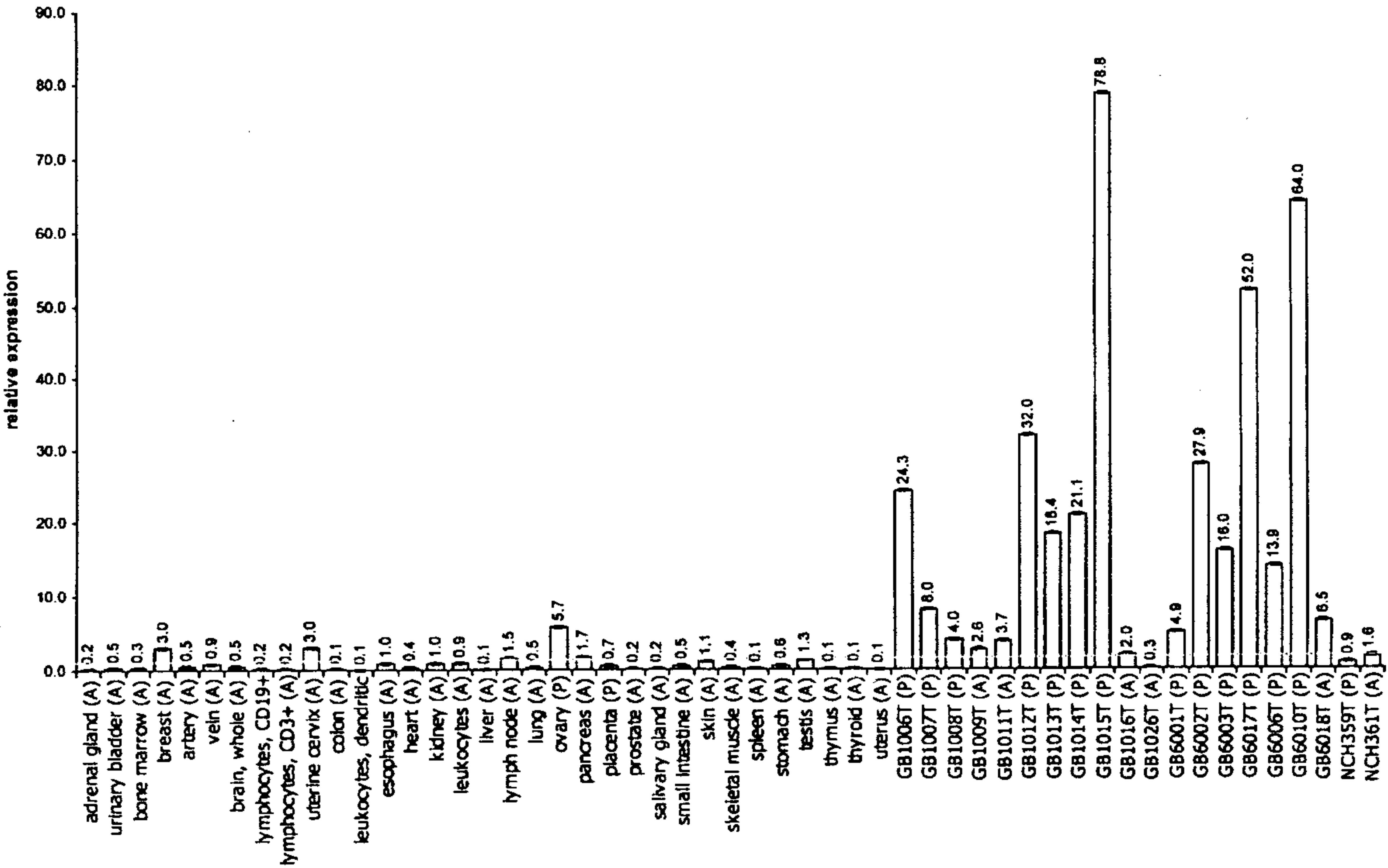
b) IGF2BP3 (Probeset ID: 216493_s_at)
