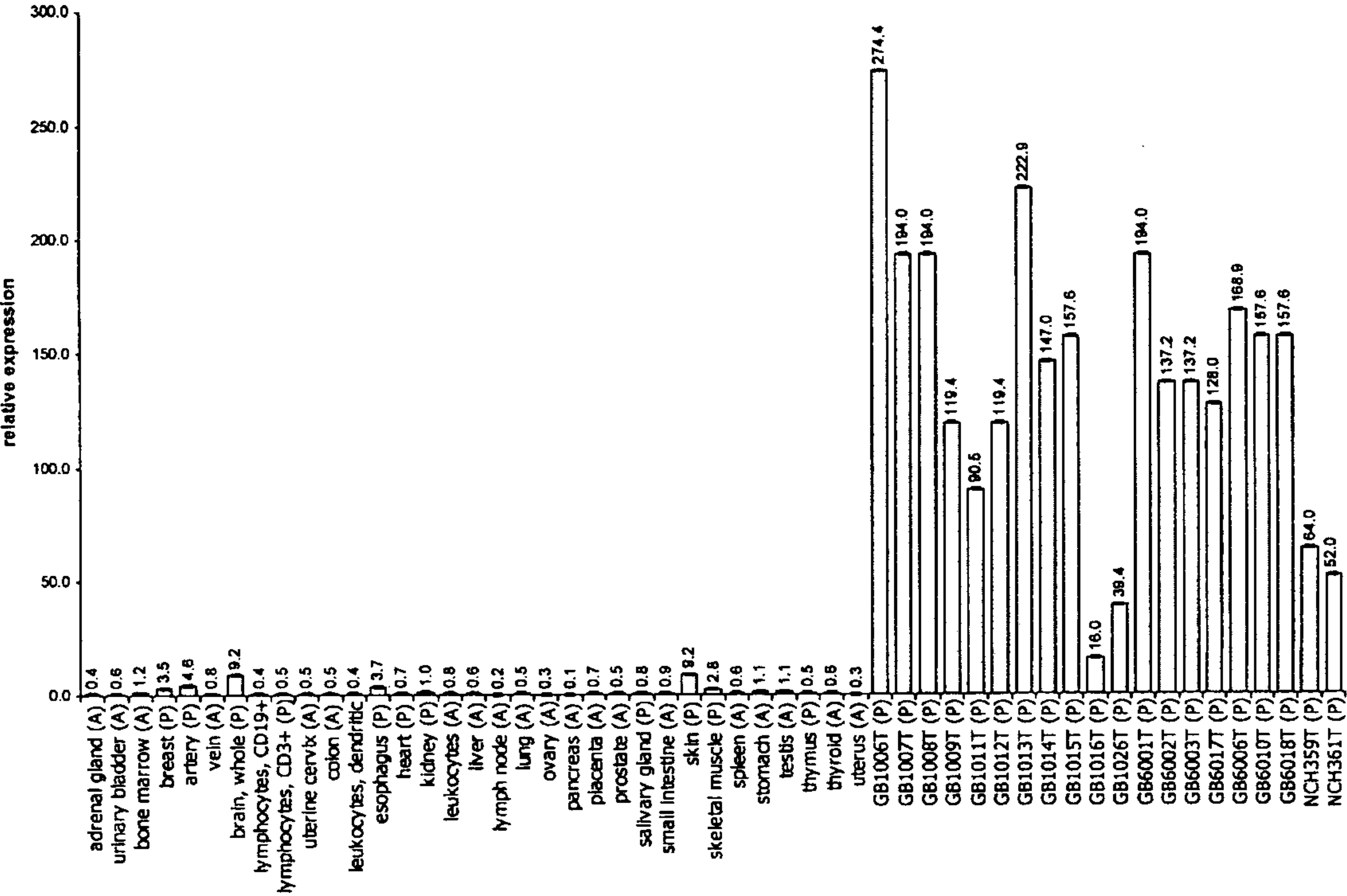
a) FABP7 (Probeset ID: 205030_at)
