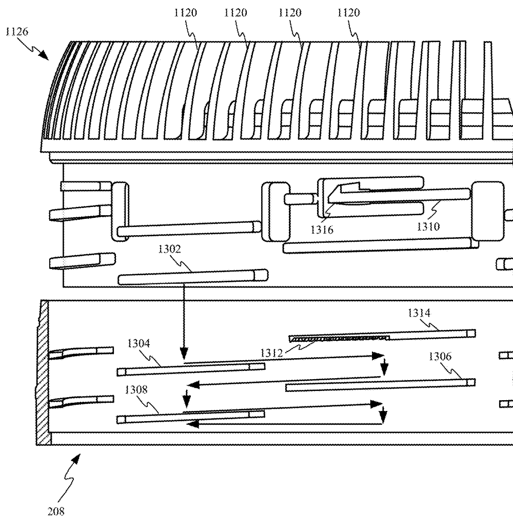
FIG. 13A
