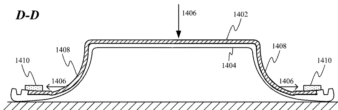
FIG. 14C
