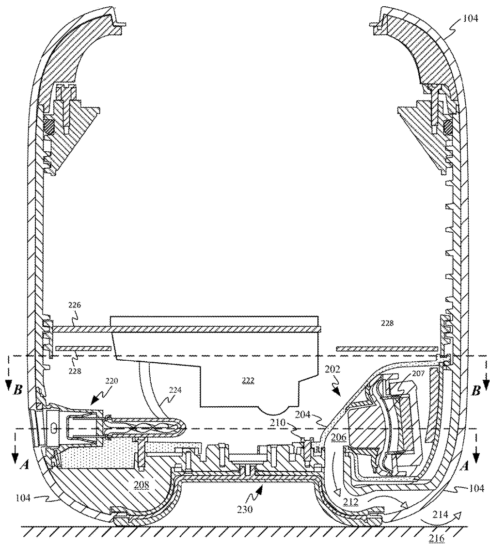
FIG. 2A
