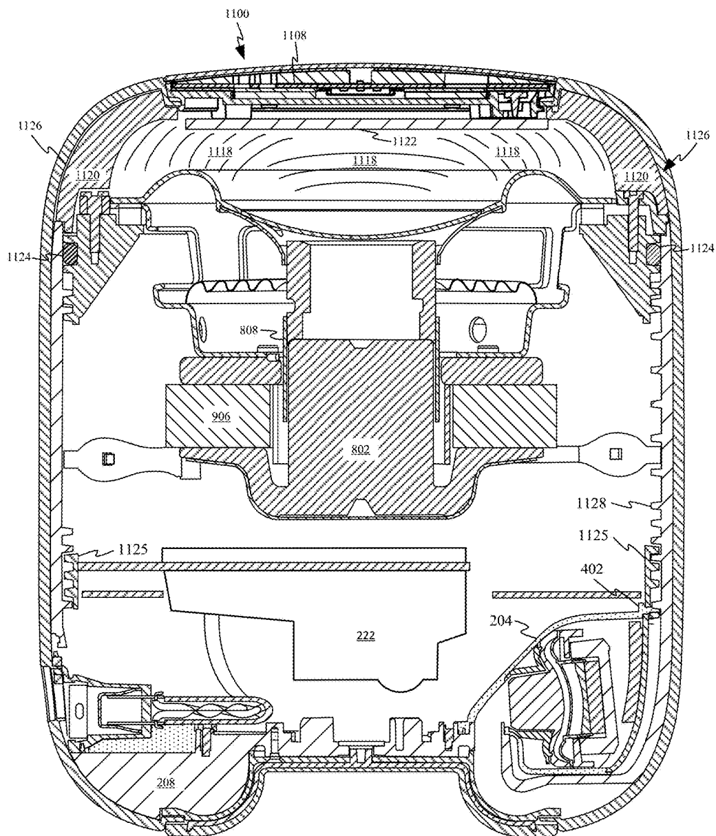
FIG. 11C
