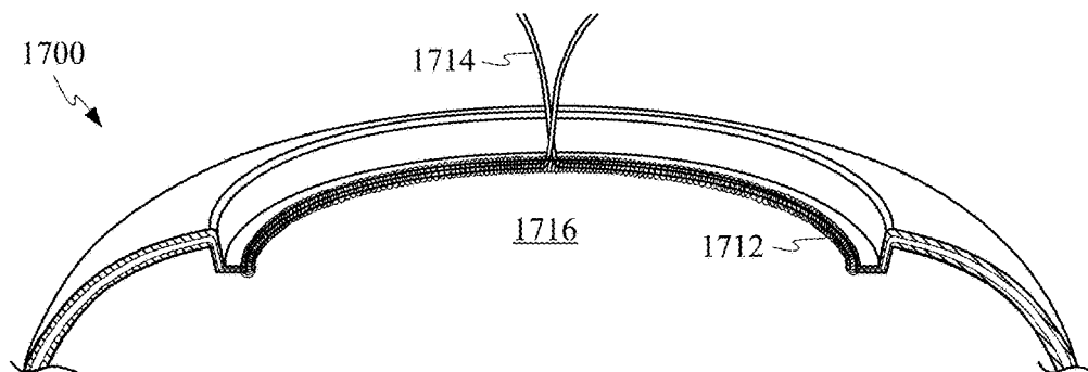
FIG. 17B
