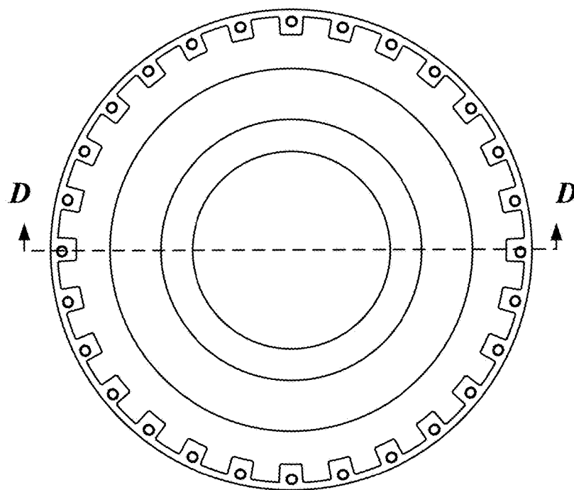
FIG. 14C
