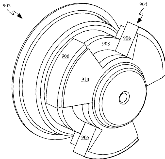
FIG. 9C
