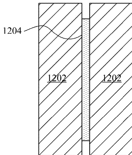
FIG. 12B
