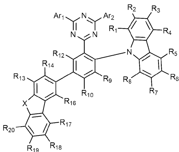
[화학식 1-8]
