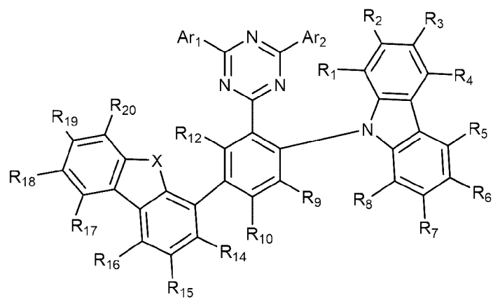
[화] 화학식 1-6]
