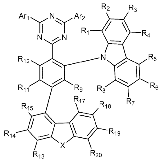
[화] 화학식 1-5]
