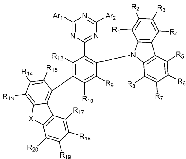
[화학식 1-8]
