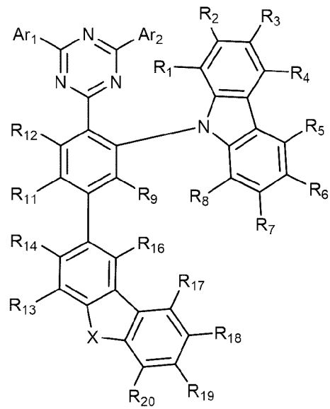
[화] 화학식 1-4]
