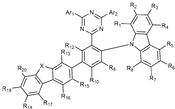
[화학식 1-7]
