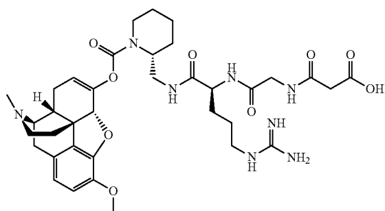
KC-31
