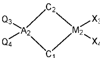
[Formule chimique 2]
