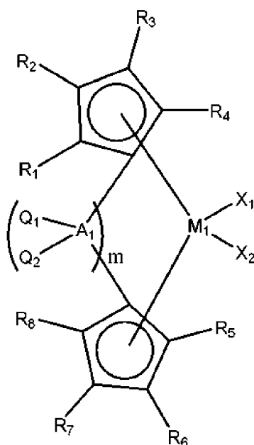
[Formule chimique 1]
