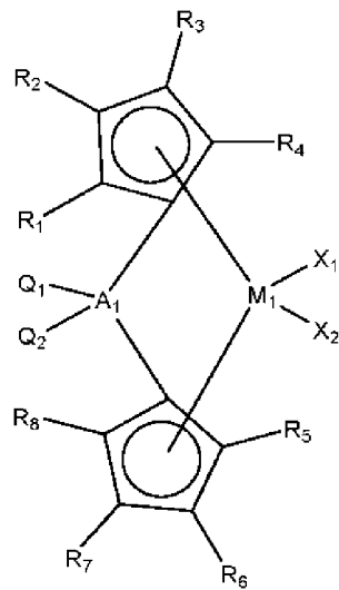
[Formule chimique 1-2]
