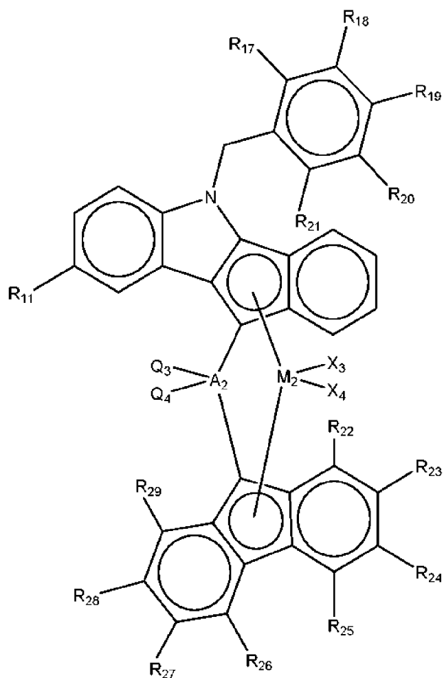
[Formule chimique 2-1]
