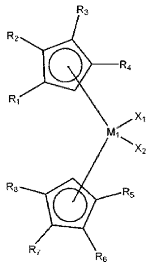
[Formule chimique 1-2]
