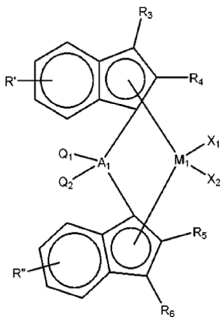
[Formule chimique 1-4]
