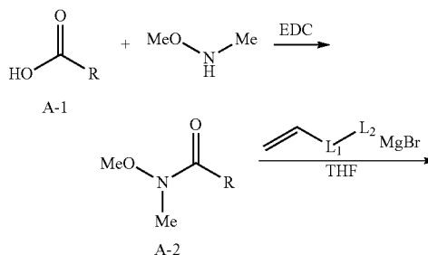
Scheme A-1
