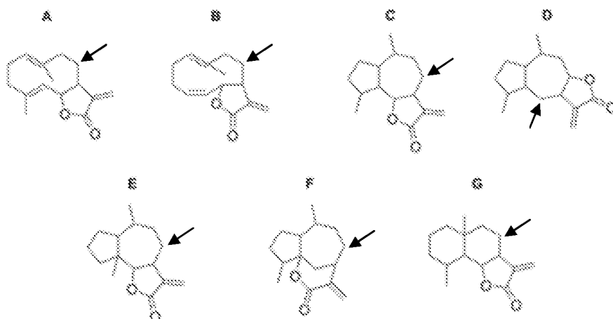
A: Germacranolides, B: Heliangolides, C+D: Guaianolides, E: Pseudoguaianolides, F: Hypocretenolides, G: Eudesmanolides.
