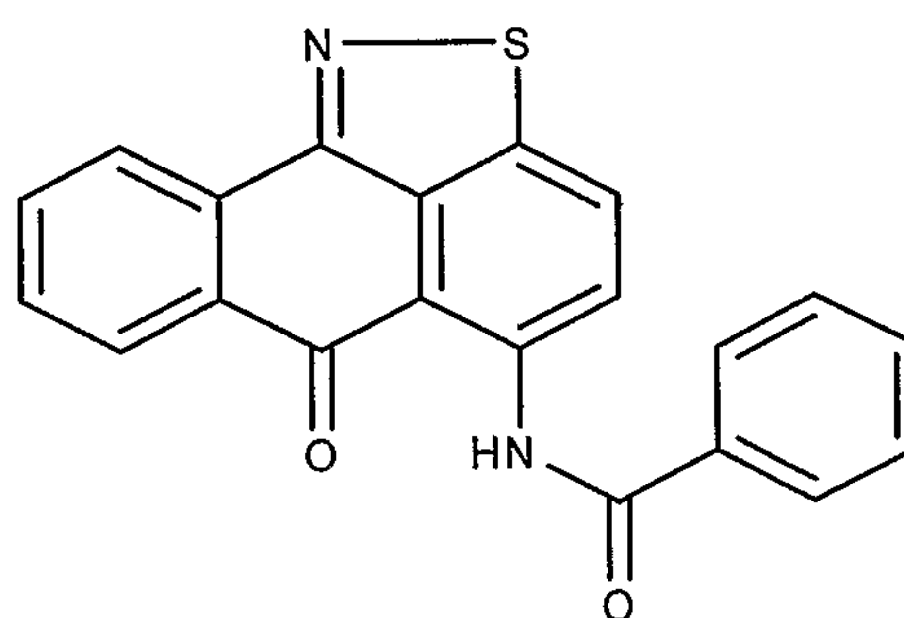
N -(6-Oxo-6 H -anthra[9,1- cd ]isothiazol-5- yl)-benzamide ;
