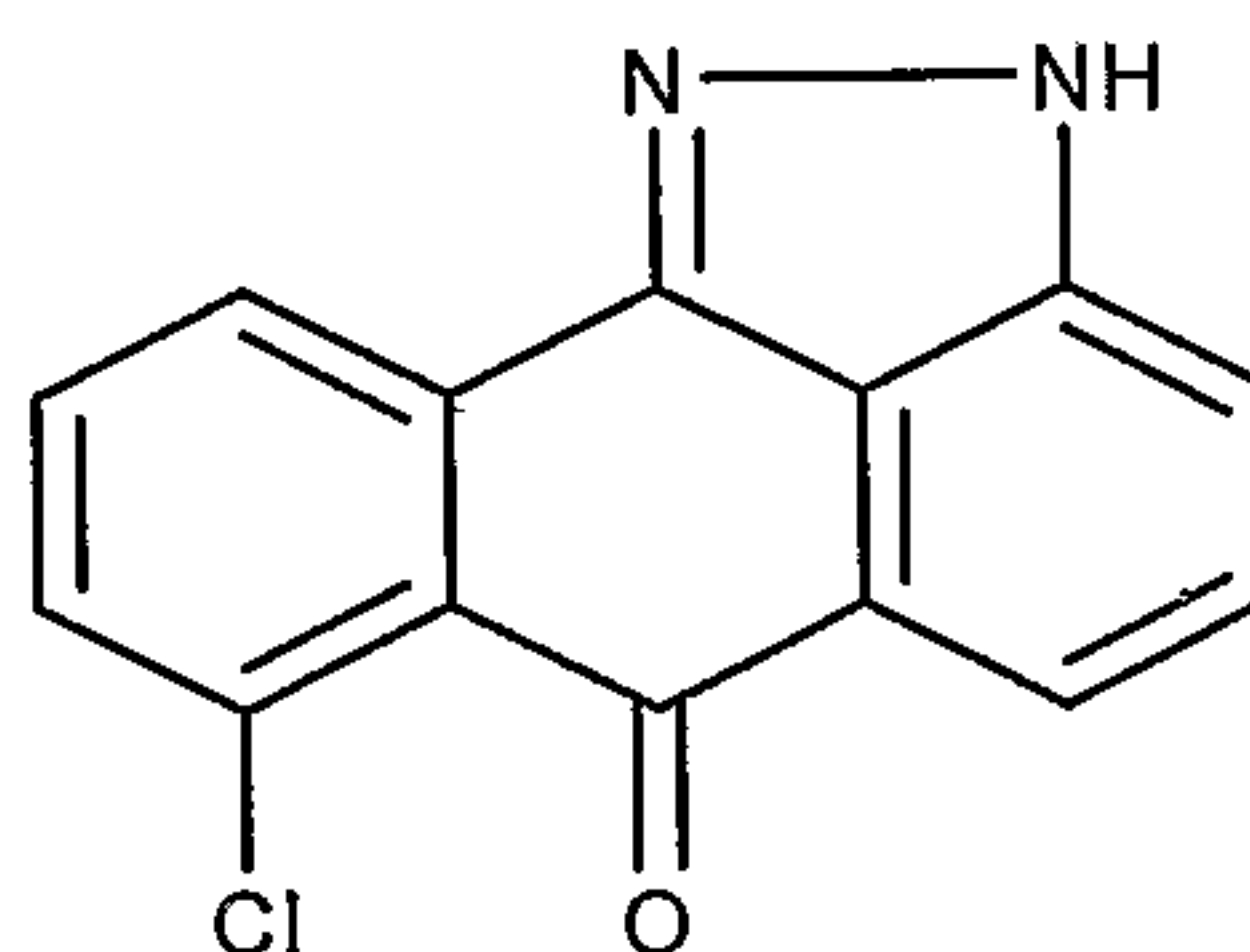
7-Chloro-2 H -dibenzo[ cd,g ] indazol-6-one ;
