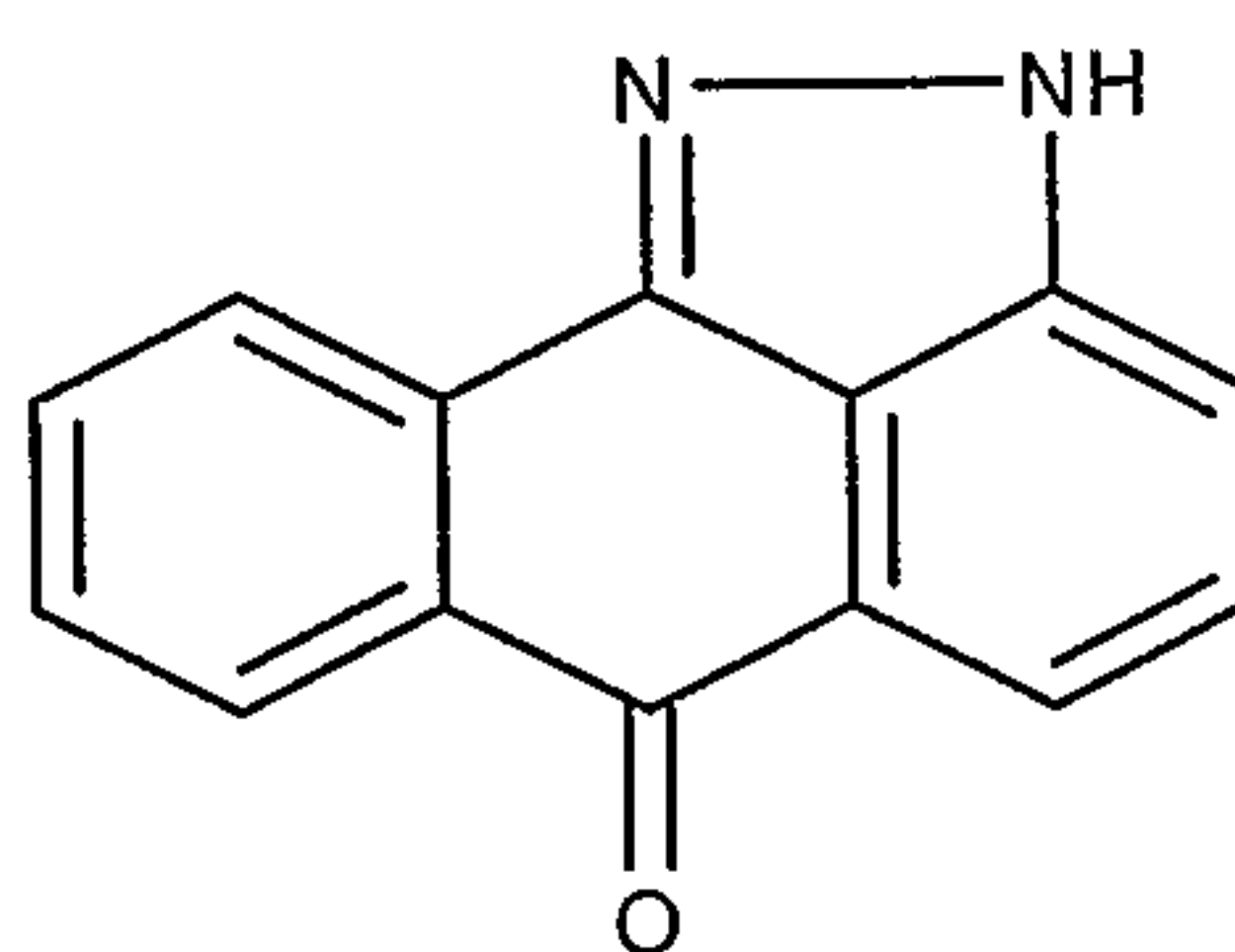
2 H -Dibenzo[ cd,g ] indazol-6-one ;
