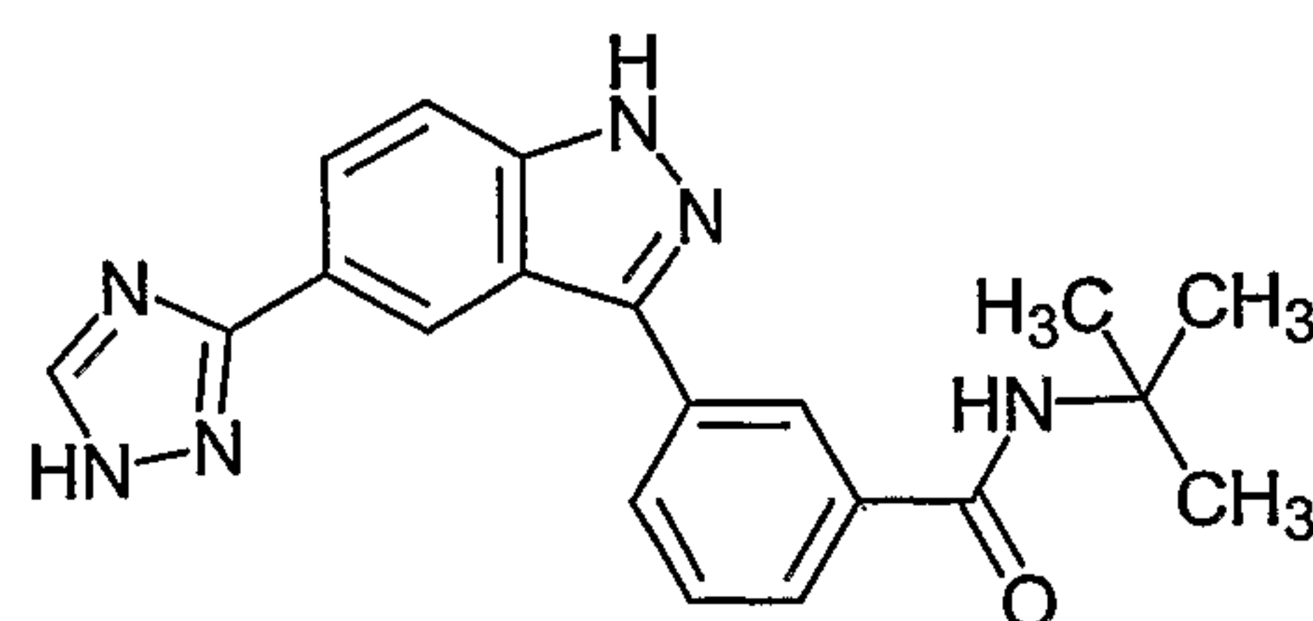
N -tert-Butyl-3-[5-(1 H -[1,2,4]triazol-3-yl)-1 H - indazol-3-yl]-benzamide ;
