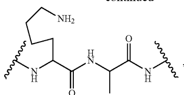
lysine-alanine (lys-ala)
