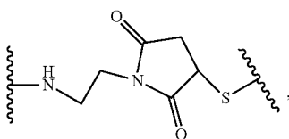
maleimidoethyl (ME)
