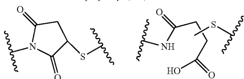
thio-maleido
