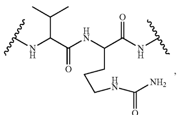
valine-citrulline (val-cit)
