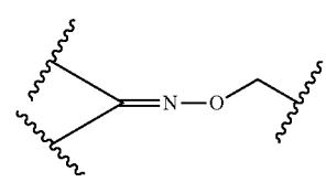
oxime
