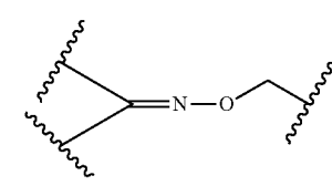
oxime
