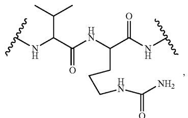
valine-citrulline (val-cit)
