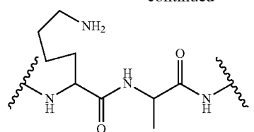
lysine-alanine (lys-ala)
