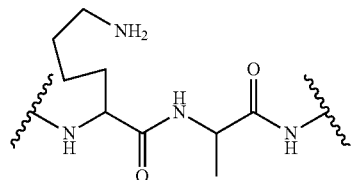
lysine-alanine (lys-ala)
