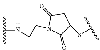
maleimidoethyl (ME)
