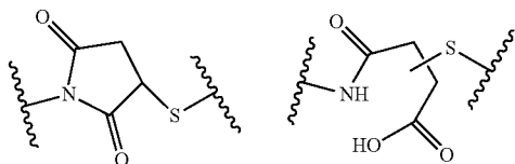
thio-maleido
