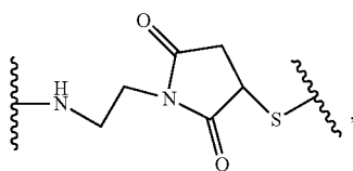
maleimidoethyl (ME)
