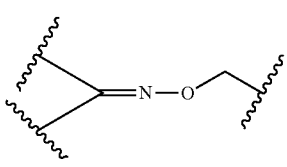
oxime
