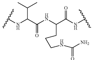
valine-citrulline (val-cit)
