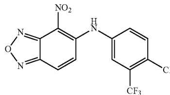
N-(4-chloro-3-(trifluoromethyl)phenyl)-4-nitrobenzo[c][1,2,5]oxadiazol-5-amine
