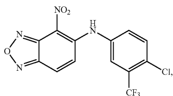
N-(4-chloro-3-(trifluoromethyl)phenyl)-4-nitrobenzo[c][1,2,5]oxadiazol-5-amine
