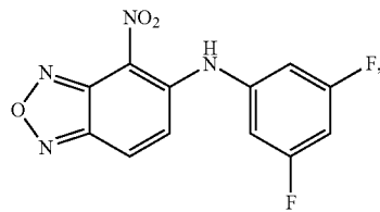
N-(3,5-difluorophenyl)-4-nitrobenzo[c][1,2,5]oxadiazol-5-amine
