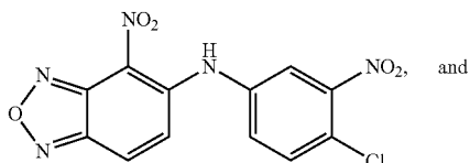
N-(4-chloro-3-nitrophenyl)-4-nitrobenzo[c][1,2,5]oxadiazol-5-amine
