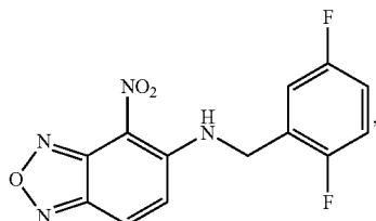
N-(2,5-difluorobenzyl)-4-nitrobenzo[c][1,2,5]oxadiazol-5-amine
