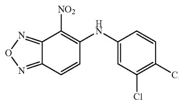
N-(3,4-dichlorophenyl)-4-nitrobenzo[c][1,2,5]oxadiazol-5-amine
