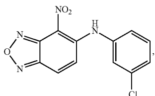
N-(3-chlorophenyl)-4-nitrobenzo[c][1,2,5]oxadiazol-5-amine
