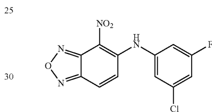
N-(3-chloro-5-fluorophenyl)-4-nitrobenzo[c][1,2,5]oxadiazol-5-amine
