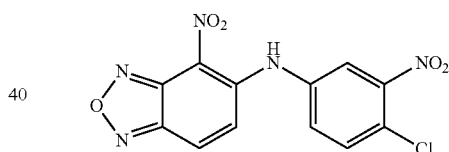
N-(4-chloro-3-nitrophenyl)-4-nitrobenzo[c][1,2,5]oxadiazol-5-amine
