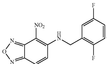
N-(2,5-difluorobenzyl)-4-nitrobenzo[c][1,2,5]oxadiazol-5-amine
