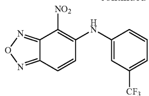
4-nitro-N-(3-(trifluoromethyl)phenyl)benzo[c][1,2,5]oxadiazol-5-amine
