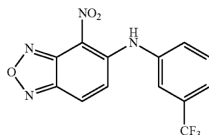
4-nitro-N-(3-(trifluoromethyl)phenyl)benzo[c][1,2,5]oxadiazol-5-amine
