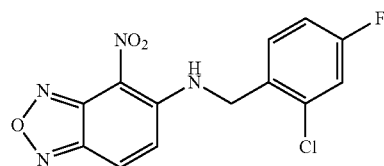
N-(2-chloro-4-fluorobenzyl)-4-nitrobenzo[c][1,2,5]oxadiazol-5-amine
