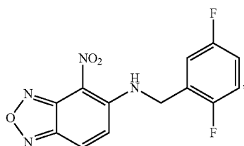
N-(2,5-difluorobenzyl)-4-nitrobenzo[c][1,2,5]oxadiazol-5-amine
