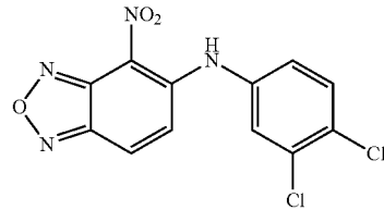
N-(3,4-dichlorophenyl)-4-nitrobenzo[c][1,2,5]oxadiazol-5-amine
