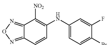
N-(4-bromo-3-fluorophenyl)-4-nitrobenzo[c][1,2,5]oxadiazol-5-amine
