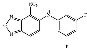
N-(3,5-difluorophenyl)-4-nitrobenzo[c][1,2,5]oxadiazol-5-amine
