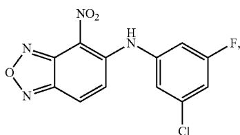
N-(3-chloro-5-fluorophenyl)-4-nitrobenzo[c][1,2,5]oxadiazol-5-amine
