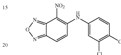
N-(3,4-dichlorophenyl)-4-nitrobenzo[c][1,2,5]oxadiazol-5-amine
