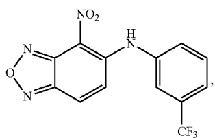
4-nitro-N-(3-(trifluoromethyl)phenyl)benzo[c][1,2,5]oxadiazol-5-amine
