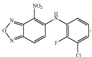
N-(3-chloro-2-fluorophenyl)-4-nitrobenzo[c][1,2,5]oxadiazol-5-amine
