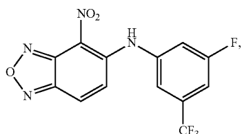
N-(3-fluoro-5-(trifluoromethyl)phenyl)-4-nitrobenzo[c][1,2,5]oxadiazol-5-amine
