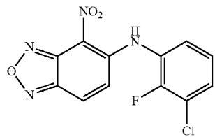
N-(3-chloro-2-fluorophenyl)-4-nitrobenzo[c][1,2,5]oxadiazol-5-amine
