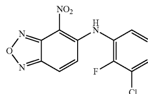
N-(3-chloro-2-fluorophenyl)-4-nitrobenzo[c][1,2,5]oxadiazol-5-amine
