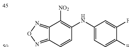
N-(4-bromo-3-fluorophenyl)-4-nitrobenzo[c][1,2,5]oxadiazol-5-amine
