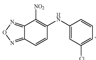
N-(3-chlorophenyl)-4-nitrobenzo[c][1,2,5]oxadiazol-5-amine
