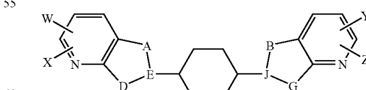
(X-7)
