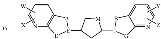
(X-3)
