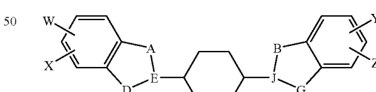
(X-6)
