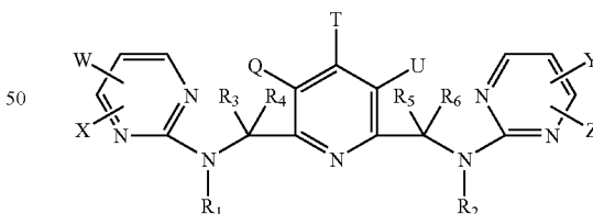
(V-4)
