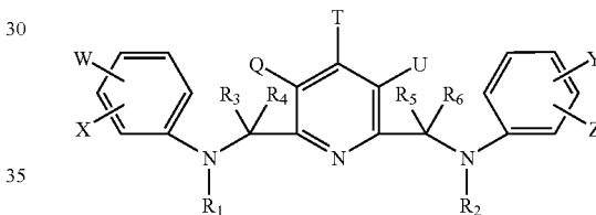
(V-2)
