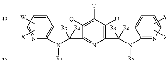
(V-3)
